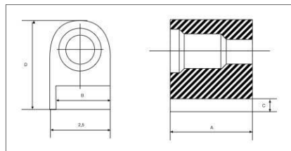
Cierre de aro de 3.5
