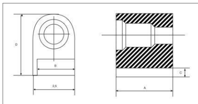
Cierre de aro de 3.3
