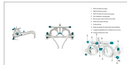
Gafa de prueba universal
